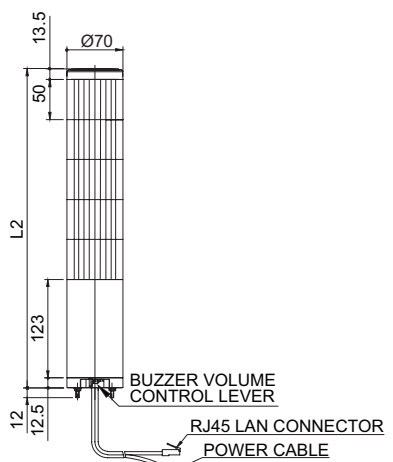
QTC(A)70ML-ETN-BZ
